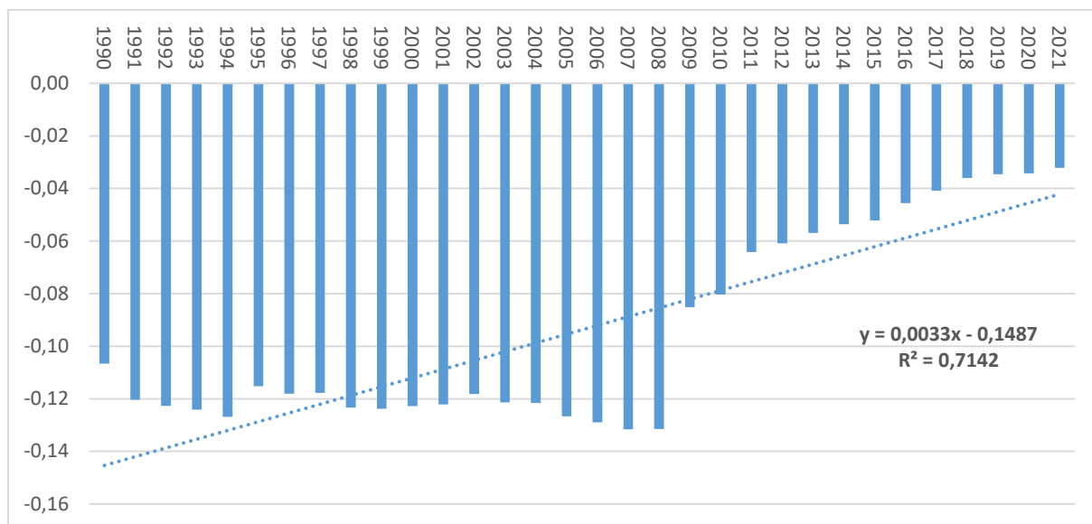
Obrázok 4: Znáznornenie rozdielu v záchytoch emisií (Gg) v kategórii 4.C Trávne porasty podľa metodiky IPCC 2006 GL (AR4) a IPCC 2019 Refinement (AR5)
