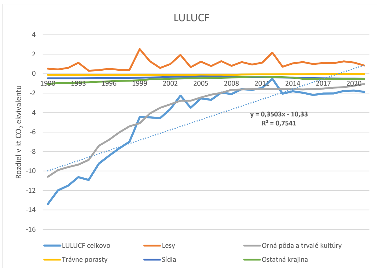
Obrázok 5: Znáznornenie celkového rozdielu v záchytoch (Gg) v LULUCF (modrá) podľa metodiky IPCC 2006 GL (AR4) a IPCC 2019 Refinement (AR5) a rozdielov podľa jednotlivých pod-kategórií
