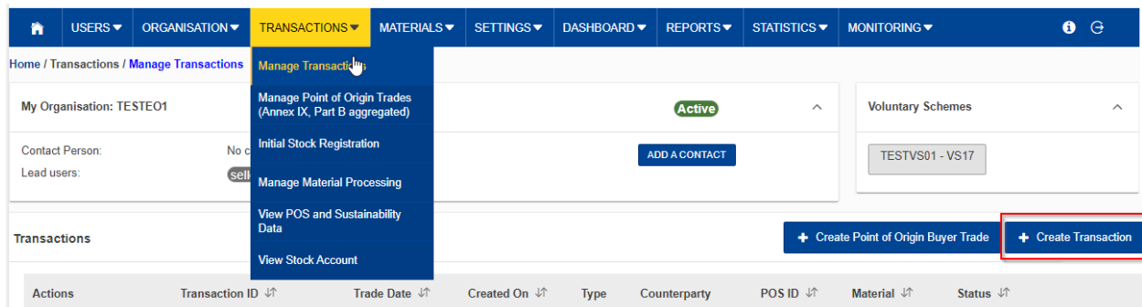
Obr 2. Vytvorenie transakcie
